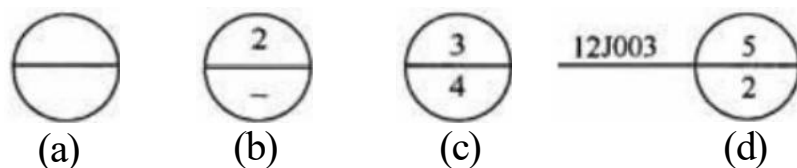
图4.6.2-2 索引符号应用示例
