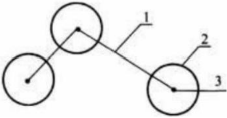
图4. 5. 2-1 初步设计和施工图设计图纸中单株种植植物标注 1—种植点连线；2—种植图例； 3—序号、树种和数量
