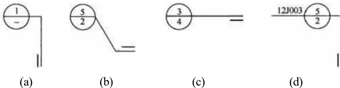
图4.6.2-3 用于索引剖面详图的索引符号
