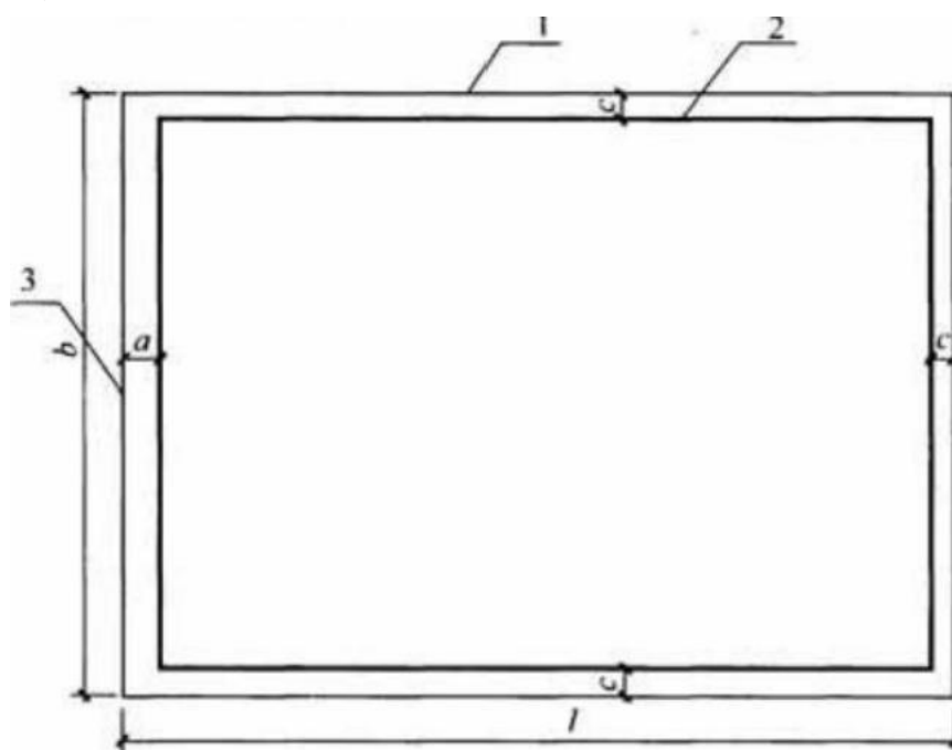
图 2.0.2 图纸图幅及图框尺寸示意
