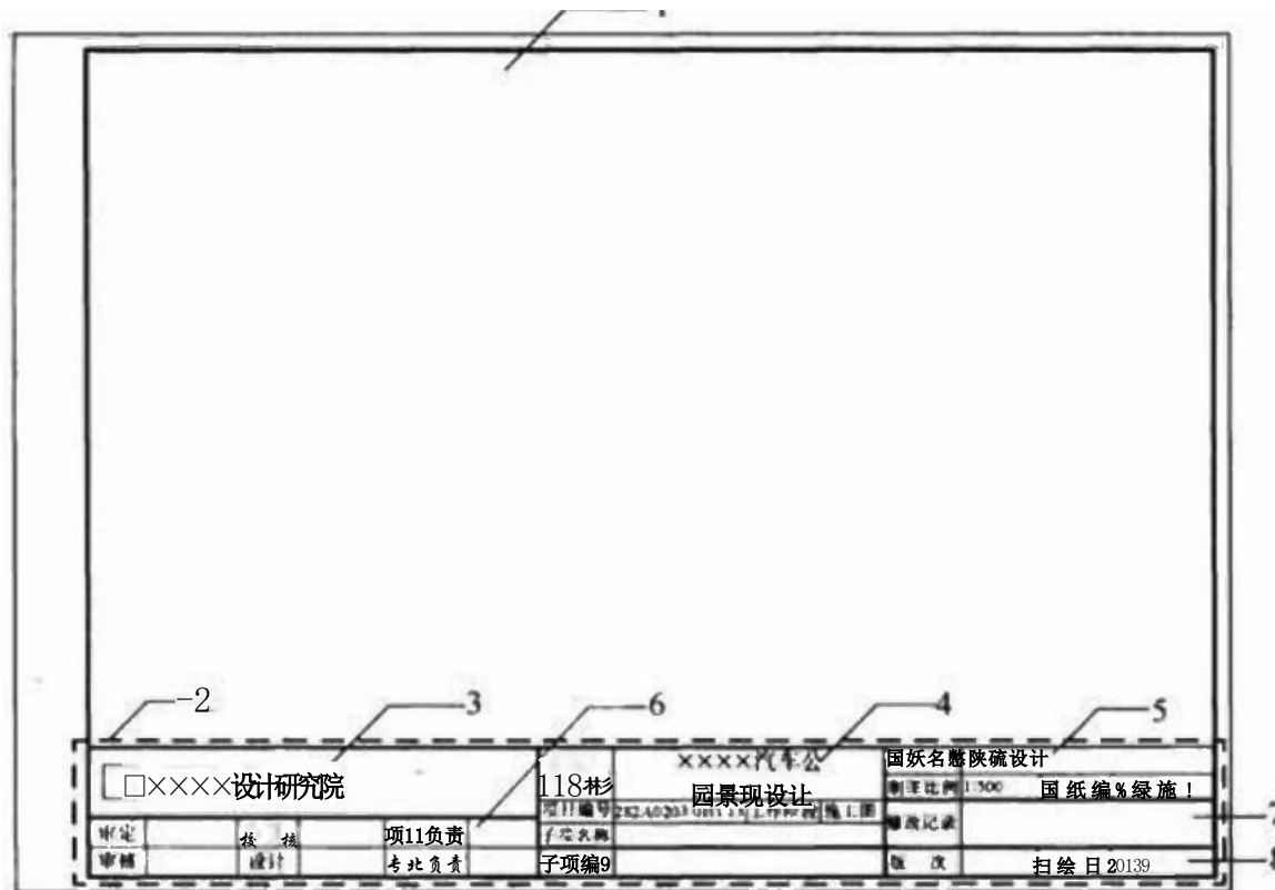
图4.1.3-2 下侧图签栏
